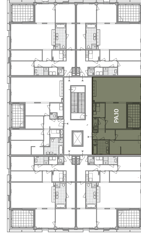
Tweede woonlaag
